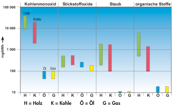
Abb. 2: Emissionen von Hausbrandfeuerungen sind brennstoffabhängig. Im Bild ist die vom Brennstoff abhängige, auf die erzeugte Wärmemenge bezogene Emission (Bandbreite) in Milligramm pro Kilowattstunde (mg/kWh) dargestellt.
