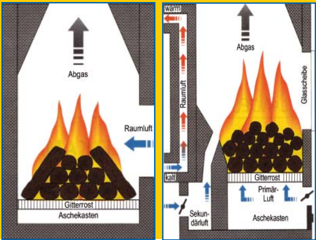
Abb. 1: Prinzipdarstellung eines offenen Kamins (links) und eines Heizkamines/Kaminofens (rechts)
